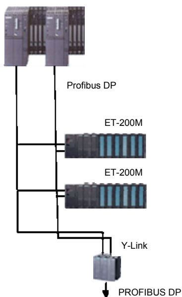
Rysunek 2. Kasety oddalonych modułów I/O – ET200M oraz moduł Y-Link – przykład połączenia.
