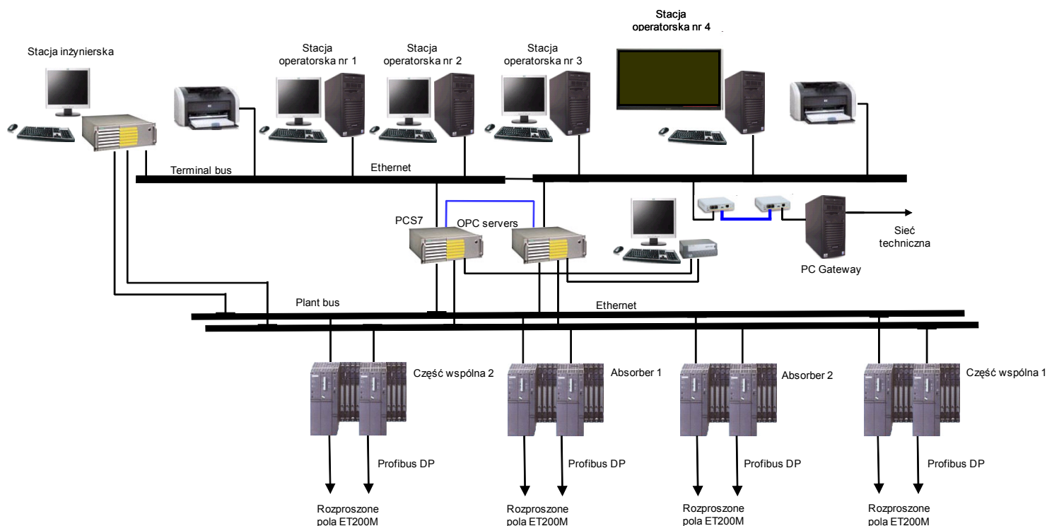
Rysunek 1. Konfiguracja systemu SIMATIC PCS7 – część centralna.
